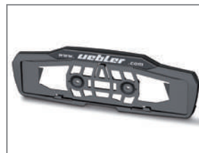
Afstandhouder 3e/4e fiets (fiets tot fiets) Afsluitbaar. Voor fietsframes van ronde buizen tot 75 mm of ovale buizen tot 75 x 45 mm. Art.nr. 19910
